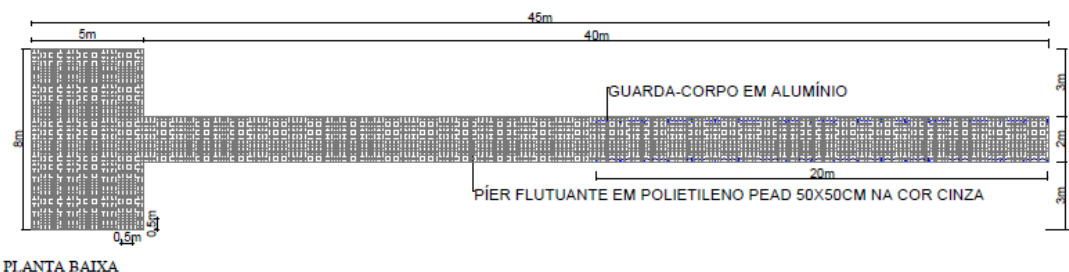
PLANTA BAIXA
