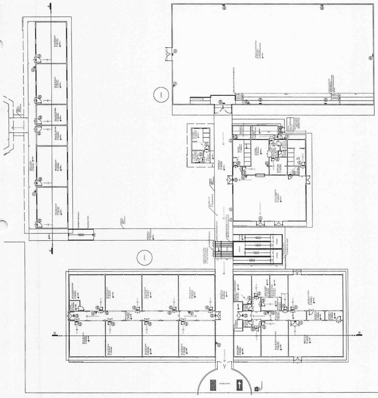
PLANTA BAIXA Escala 1:150
