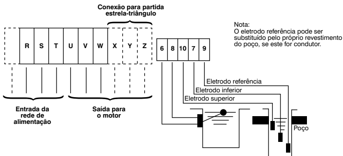
Figura 6.6 - Conexão do Quadro de Comando
