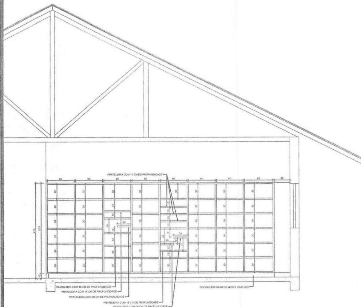
VISTA 3 ESCALA 1:50
