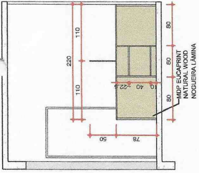
VISTA 02 - MESA POSTERIOR
