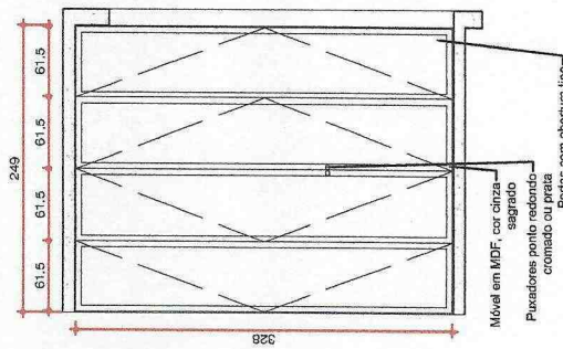
VISTA 01 - ABERTURA DAS PORTAS EXTERNAS ESC: 1/50
