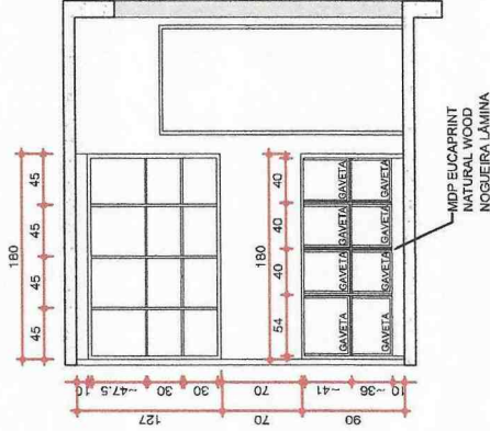
VISTA 03 - DIVISÓRIAS INTERNAS
