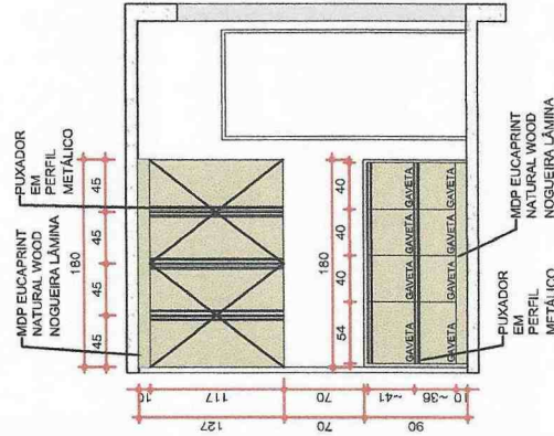
VISTA 03 - ABERTURA DAS PORTAS
