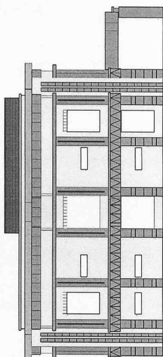
FACHADA 4 ESC: 1/100
